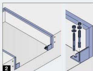
Вид сзади на модель для приямка Р, включая подъемное приспособление
