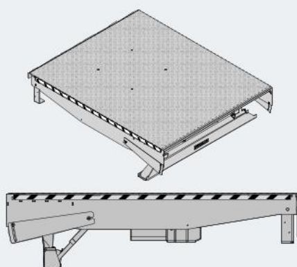
HTL 3-P в смонтированном состоянии
