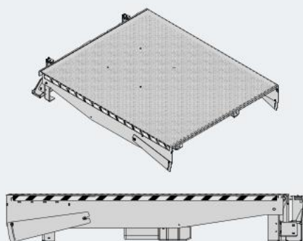
HTL 3-P в состоянии транспортировки
