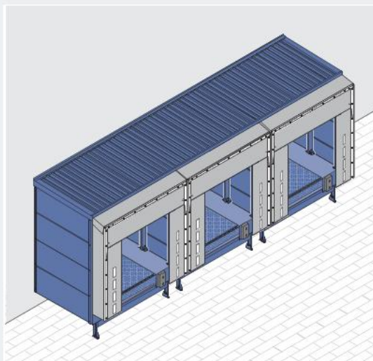
Двустенная панель 42 мм
